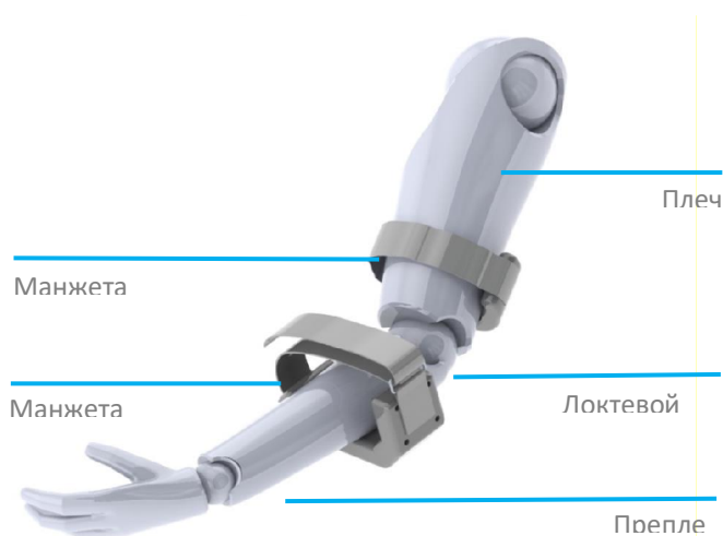
Рисунок 4 –Схема фиксации кистевой манжеты (для модели V)
